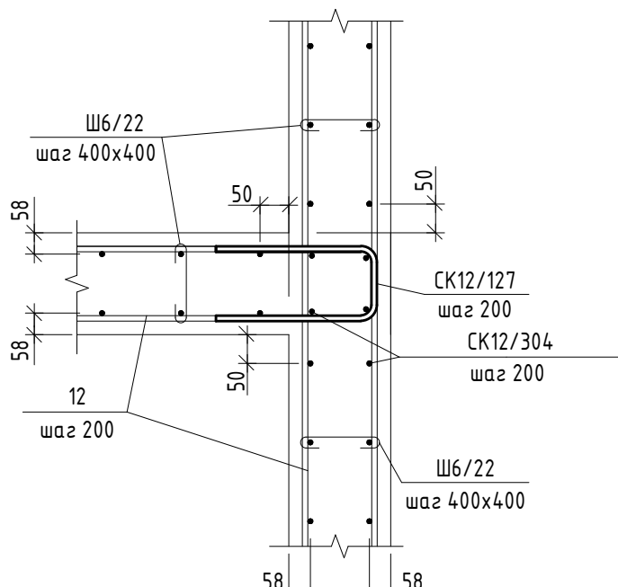
Узел Т-образного соединения стен
