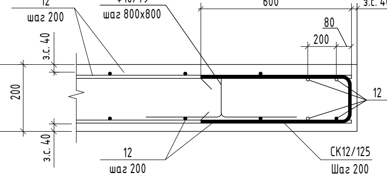
Узел Т-образного соединения стен
