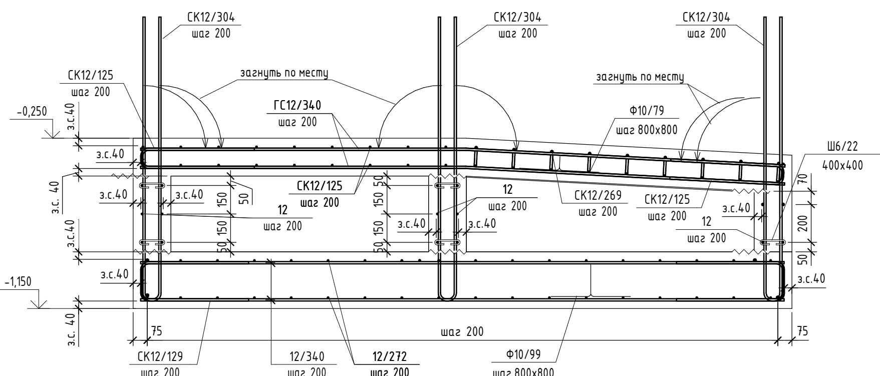
Типовой узел армирования торца фундаментной плиты
