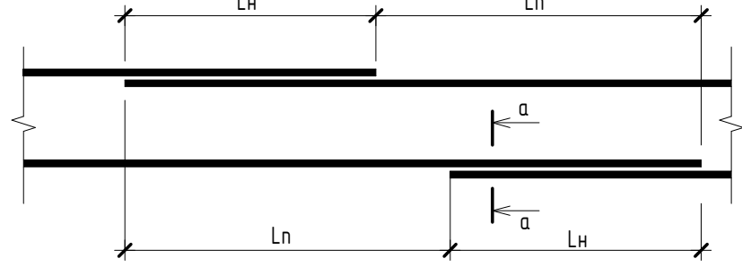
Схема стыка арматурных стержней А500С (перепуск стержней без сварки)
